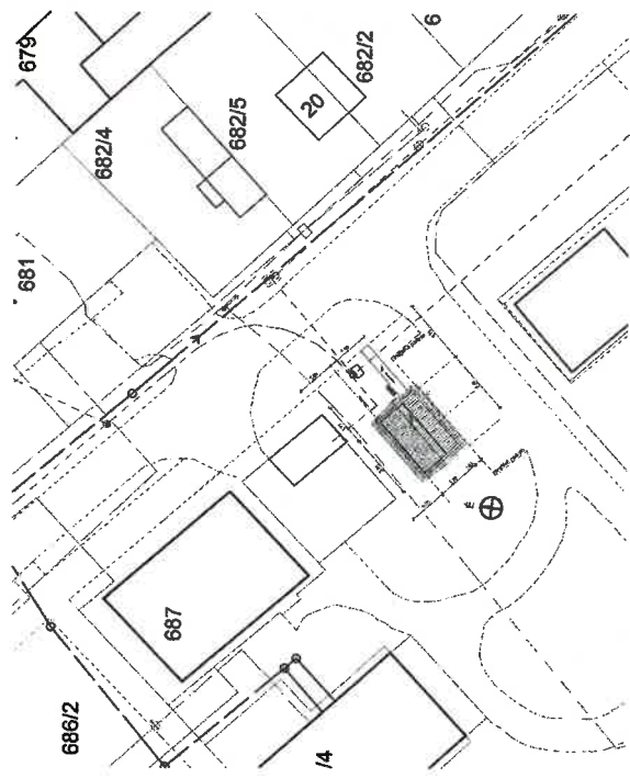
-3- HELYSZÍNRAJZ 1:500
